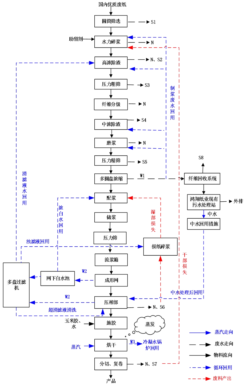
图 1 本项目生产工艺及产污节点图
